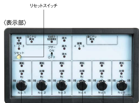
運転モード切替スイッチ
