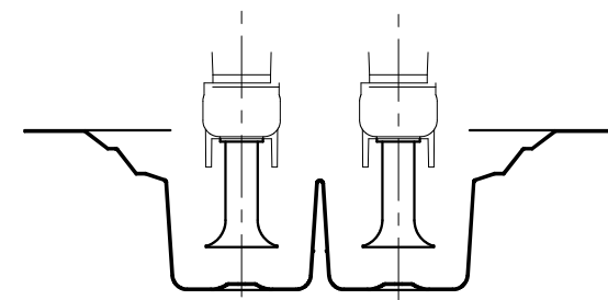
ベルマウス詳細図
