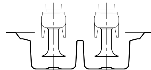
ベルマウス詳細図
