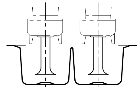
ベルマウス詳細図
