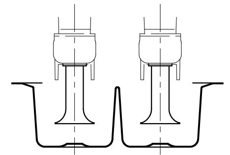
ベルマウス詳細図
