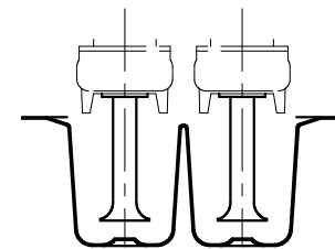
バルマウス詳細図
