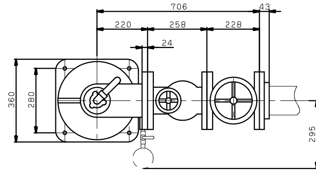
チェック弁/スルース弁付
