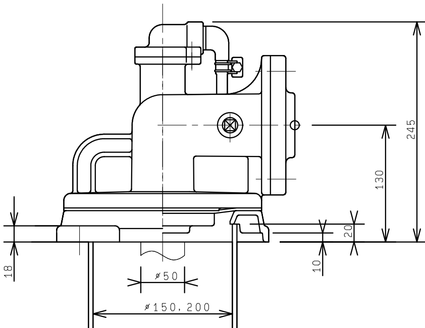
正面図
