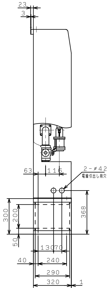
矢視A (本体下部詳細)
