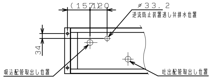
矢視A (本体下部詳細)
