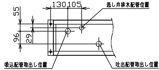
断面AA(本体下部詳細)
