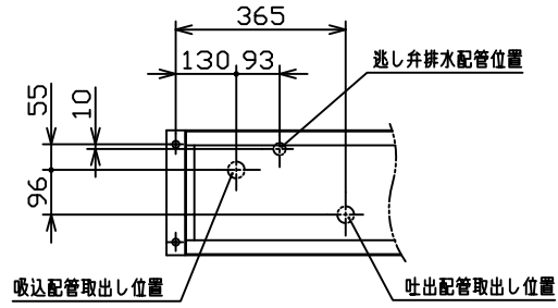
断面AA(本体下部詳細)
